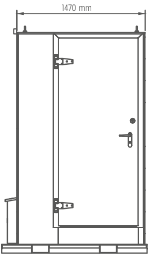
Vorderansicht
